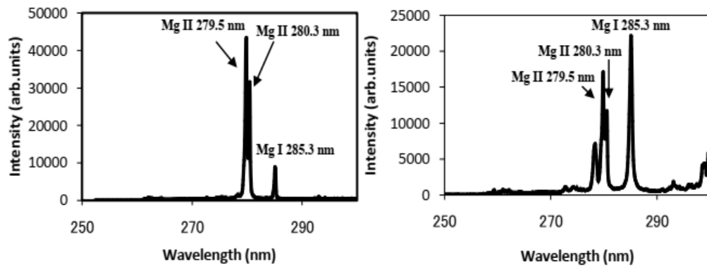
Gambar3. Spectrum emisiMg, (a) dengan laser TEA CO2, dan (b) menggunakan laser Nd:YAG
